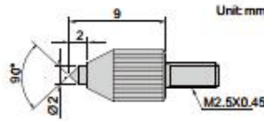
6282-0801
