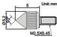
6282-0701
