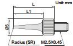
6282-1601
