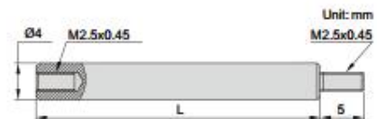
6282-2010
