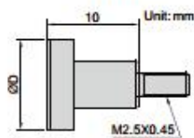
6282-1201
