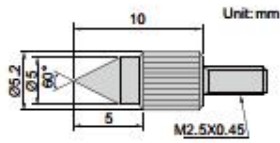
6282-0601
